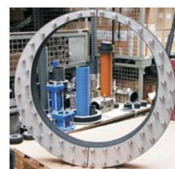
exzent. Pressringdichtung
